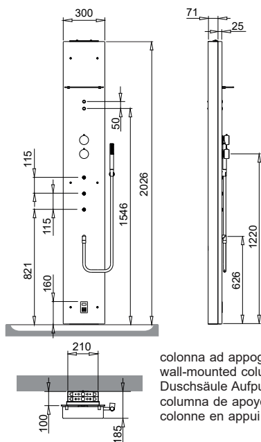
colonna ad appoggio wall-mounted column Duschsäule Aufputz columna de apoyo colonne en appui
