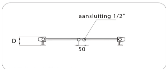
Middenaansluiting
