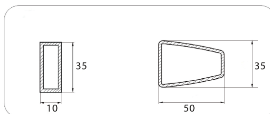
Afmeting buizen
